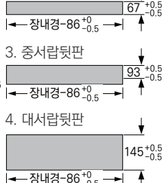
2. 속,소서랍뒷판
