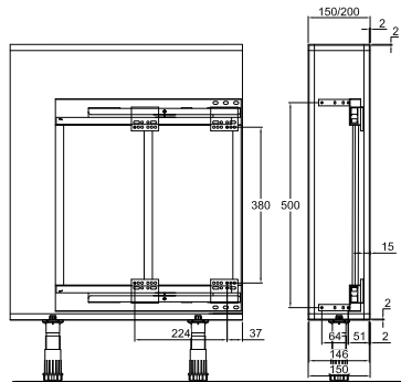
측면 보링도 (좌측용은 반대면)
