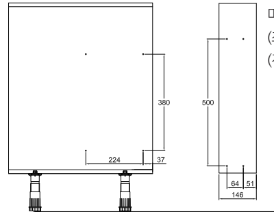
측면 보링도 (좌측용은 반대면)
