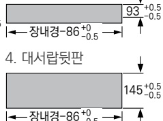
3. 중서랍뒷판
