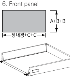
5. 속서랍 앞판 : 장내경 -80
